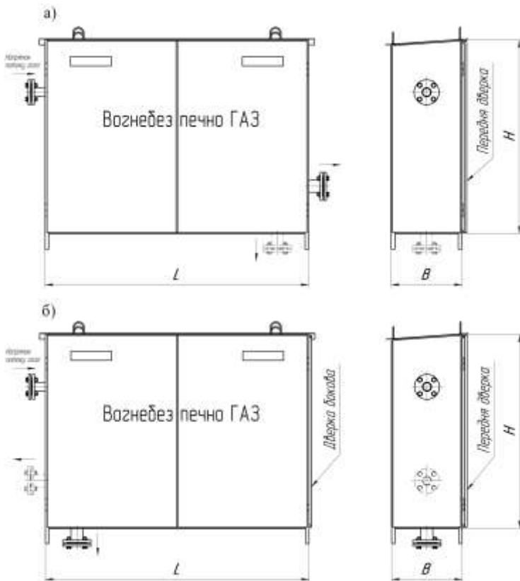
Рисунок 1 – Габаритно-приєднувальна схема газорегуляторного пункту ШГРП 50-3: а) – з однією або з двома лініями редукування; б) з однією або двома лініями редукування та вбудованим вузлом обліком газу
