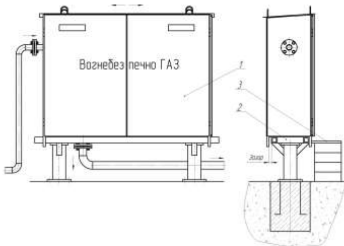
1 – газорегуляторний пункт; 2 – опорна рама; 3 – площадка обслуговування Рисунок 2 – Схема встановлення ШГРП на об'єкті
